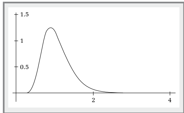
Figura 1. Función de densidad de una lognormal con \mu = 0 y \sigma^2 = 1/3 .
